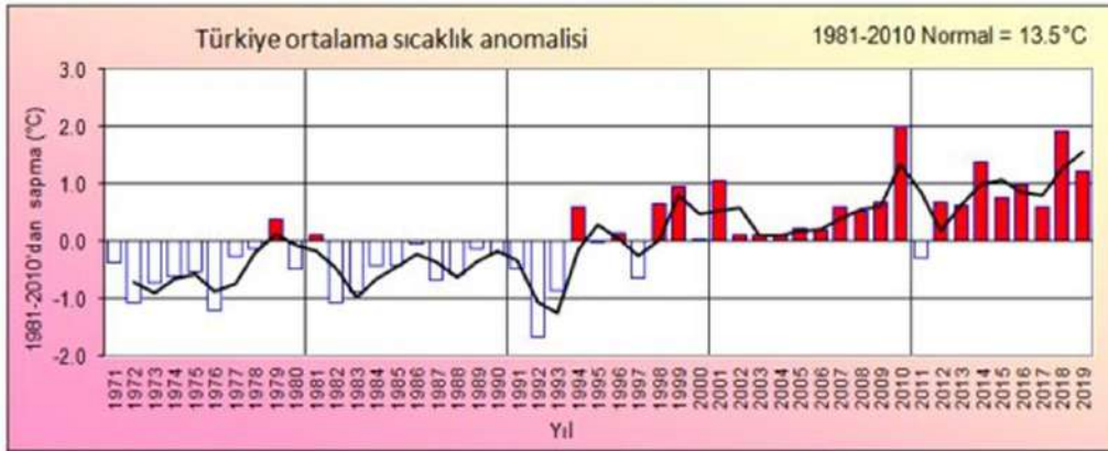
Şekil 32 Türkiye Ortalama Sıcaklık Anomalisi (Meteoroloji Genel Müdürlüğü, 2020) 14
