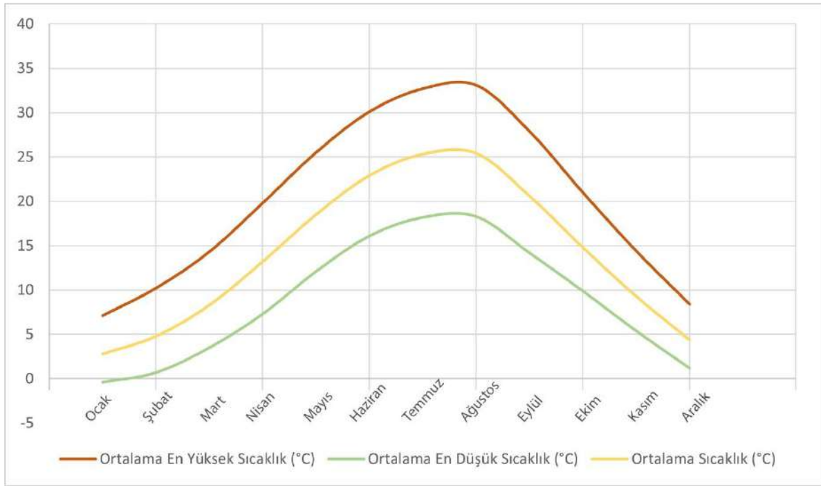
Şekil 29 Edirne Aylara Göre Sıcaklık Değerleri
