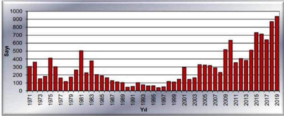
Şekil 31 Türkiye Yıllara Göre Ekstrem Hava Olayı Sayısı (Meteoroloji Genel Müdürlüğü, 2020) 13
